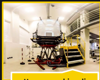
Una vera cabina di carrello elevatore
